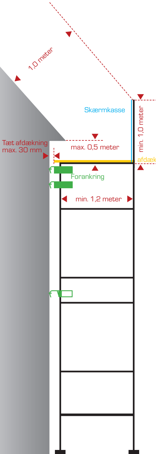
Fig. 1 Dobbelt forankring med murankre på murbukkens overligger. Monter forankring inden platforme.
